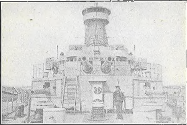
Узброєне передної части лінійного корабля.
