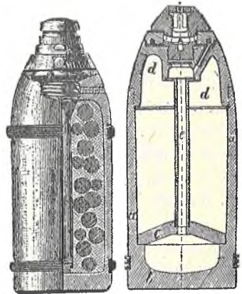
Шрапнелі: з правого боку німецький, з лівого боку швайцарський.
