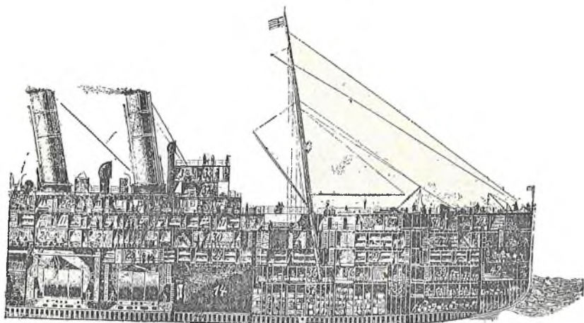
Поздовжний переріз німецького пасажирського корабля „Цісар Вільгельм I.”
