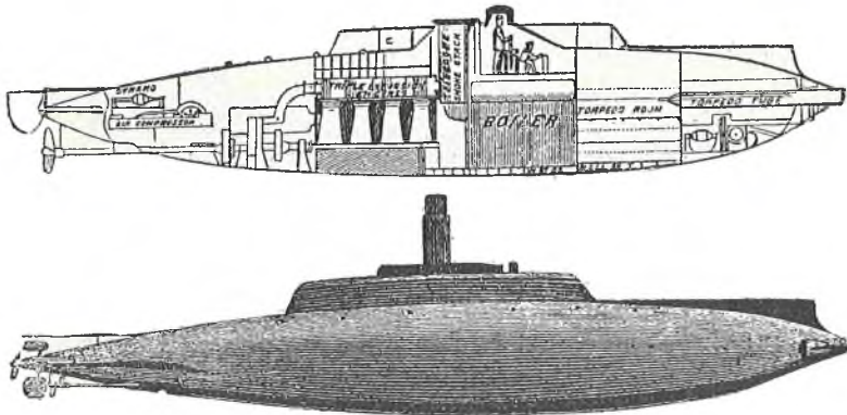
Підводне судно Голянда (перевіз і вид зверху).
