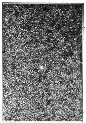
Образок 43. Застихача Молочної Дороги коло Денебу і громаді Лебедя, раз із мраківним зоряним „Америсом“ по правій стороні а зліво.
